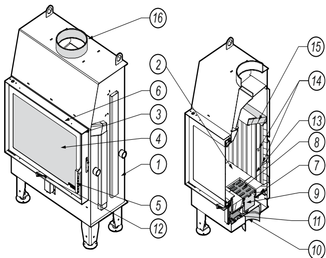
Rysunek 1. Budowa wkładu kominkowego DEFRO HOME IMPULS z drzwiami rozwieralnymi.
