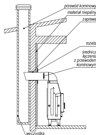
Rysunek 16. Podłączenie wkładu kominkowego do przewodu kominowego.
